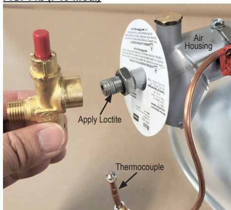
FIG. 14b (I-40-Mod.)
