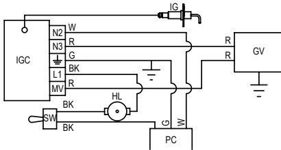
ELECTRICAL CONNECTION DIAGRAM / CONNEXIONS ÉLECTRIQUES / DIAGRAMA DE CONEXIONES ELÉCTRICAS
