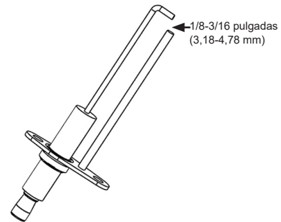
FIG. 18 SOPORTE DE MONTAJE DEL ENCENDEDOR
