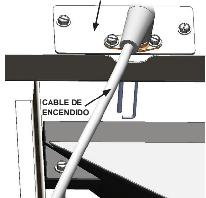
FIG. 18 SOPORTE DE MONTAJE DEL ENCENDEDOR
