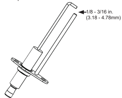
FIG. 18 SUPPORT DE MONTAGE DE L'ALLUMEUR
