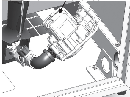
FIG. 25 ROBINET DE RÉGLAGE DU GAZ
