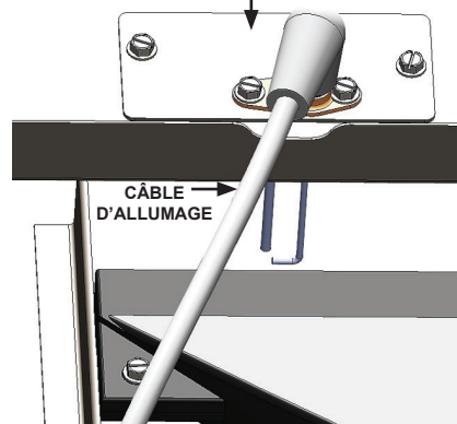
FIG. 18 SUPPORT DE MONTAGE DE L'ALLUMEUR
